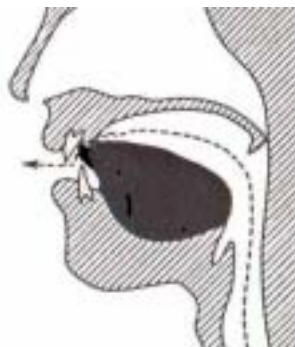
【図-9】 [ð]
