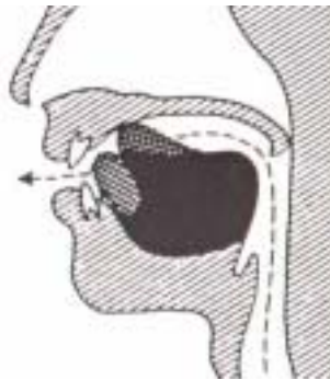
【図-18】 [r]
