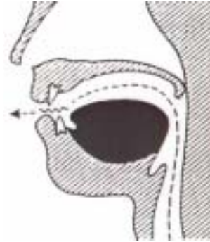
【図-3】 [β]
