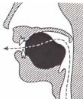
【図-14】 [ʎ]
