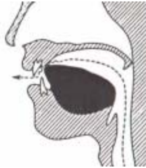
【図-6】 [s]
