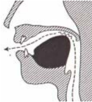
【図-12】 [x], [χ]
