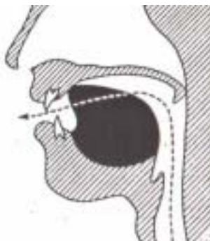
【図-13】 [l]
