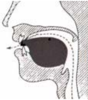
【図-5】 [θ]
