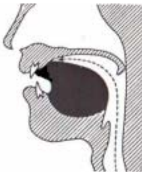
【図-8】 [d]
